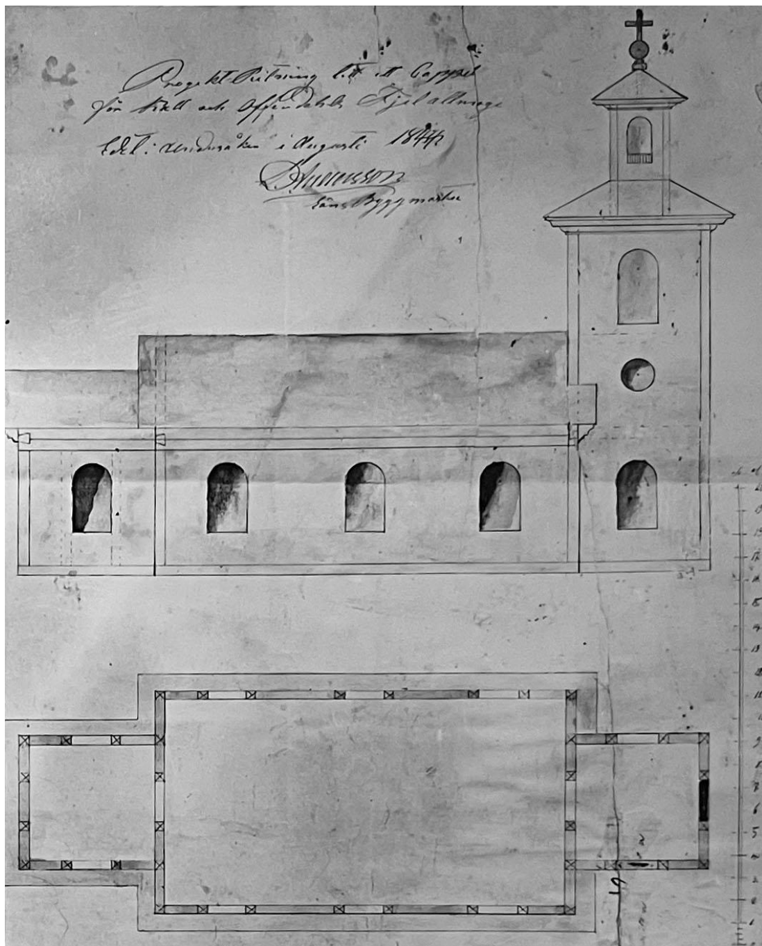
Figur 1 Ritning till Kolåsens kapell 1844 (Ejneg12186, Jamtli).
