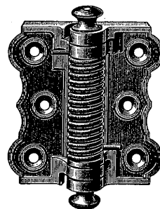
Dörrstängare N:o 5467. Automatisk fjäderstängning, enkelt och mycket billigt, men ändock fullt effektiv konstruktion. Bör ej saknas på någon dörr, som man ständigt önskar stängd. Höjd ca 10 cm. Pris 0,90 pr par.
